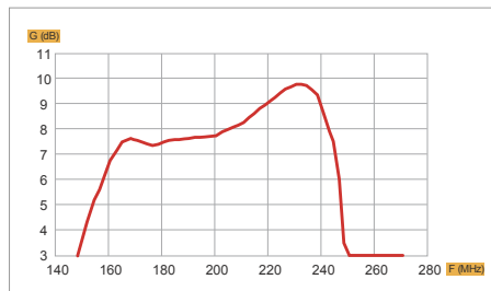
Frekventni odziv
