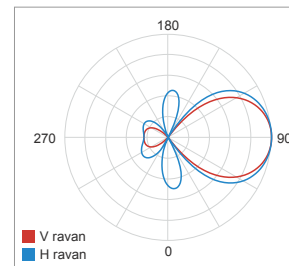
Dijagram zracenja
