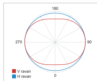
Dijagram zracenja
