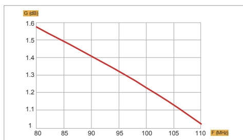
Frekventni odziv
