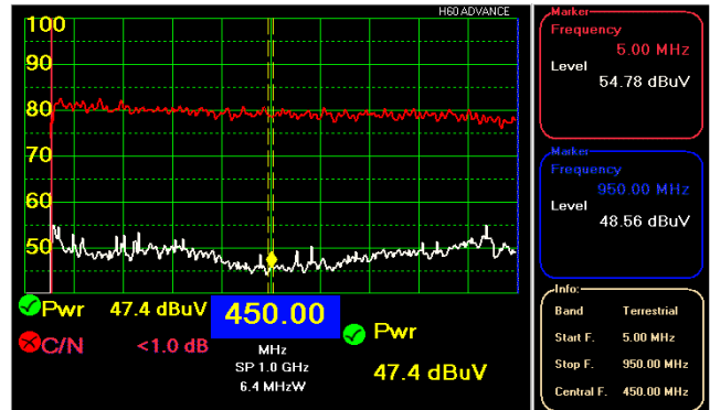
Izolacija između izlaza
