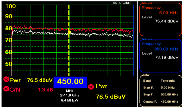
Frekventni odziv (crvenom bojom ulazni spektar, belom bojom izlazni spektar)
