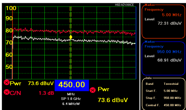
Frekventni odziv (crvenom bojom ulazni spektar, belom bojom izlaznispektar)
